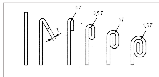
图6 - T-bends
