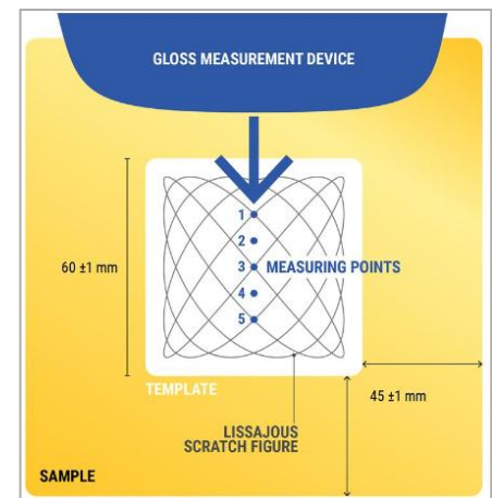
数字 9 - 样品上测量点的示意图
